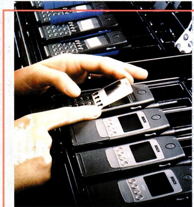
La fabrication des mobiles se fait à la chaîne (en bas à droite) mais n'est pas tout automatisée. Les interventions humaines sont fréquentes et minutieuses (en bas à gauche, la fixation de la carte de commande et ci-dessus le montage de l'écran). Usine Bosch Telecom de Pandrup (Danemark).
