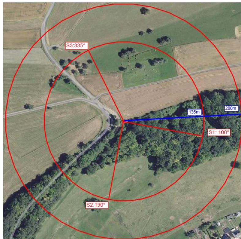
Figure 3 : Plan de la zone autour de l'antenne.
