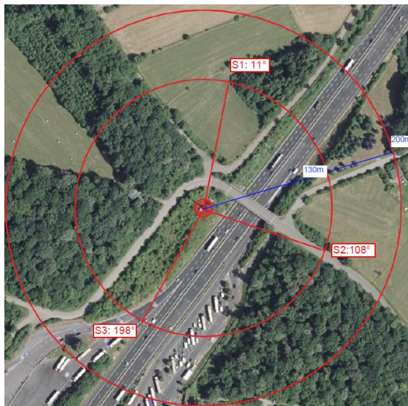
Figure 3 : Plan de la zone autour de l'antenne.
