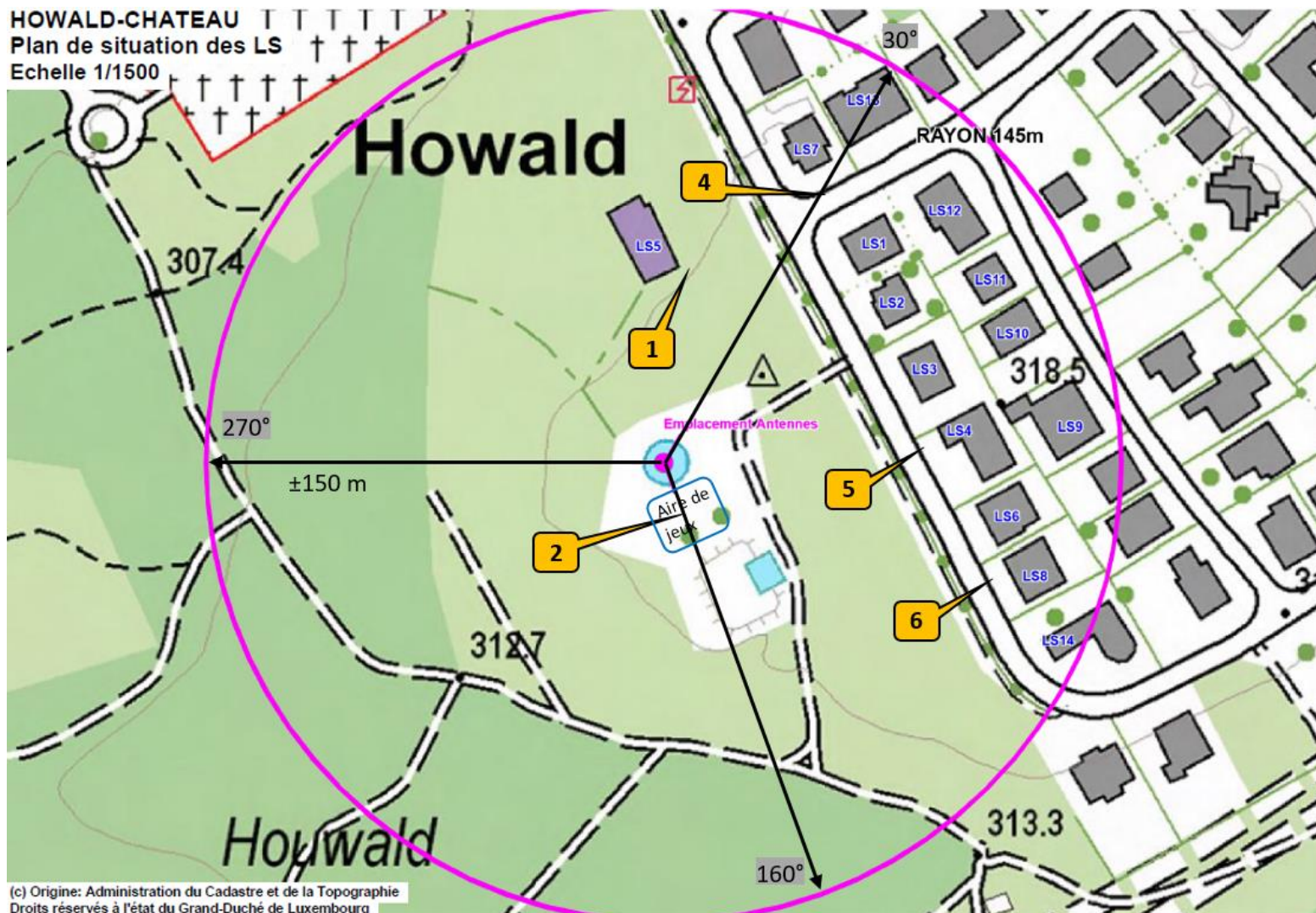
Figure 2 : Plan de la zone autour de l'antenne.
